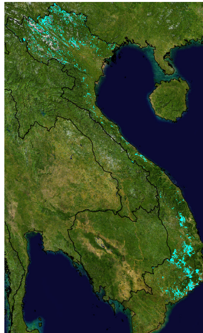
(d) max-benefit: biodiversity conservation
